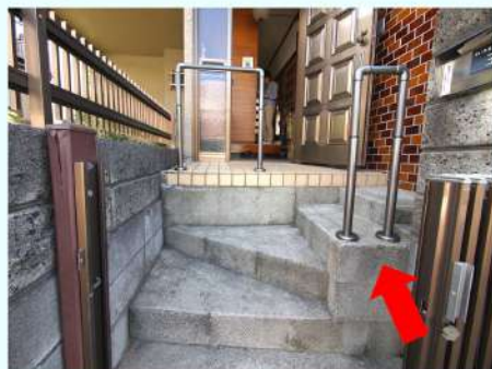
ステップの幅が狭い場所でも 設置可能です！
