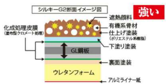
シルキーG2断面イメージ図
